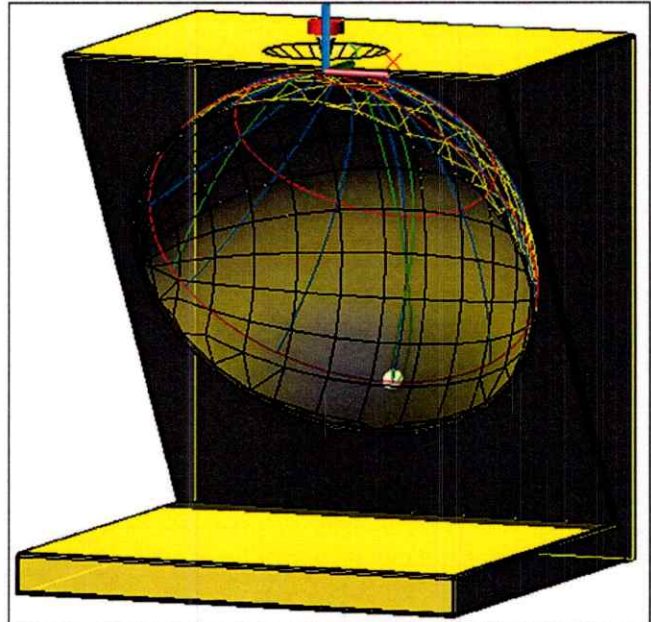
Fig. 1. Verticale scaphezonnewijzer vanuit het zuidoosten gezien.
