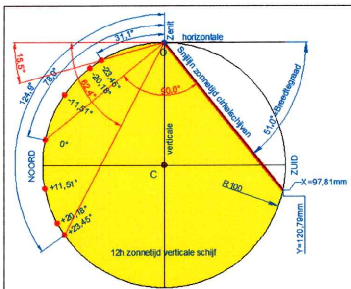
Fig. 4. 12h-zonnetijdschijf met de gemeenschappelijke snijlijn.
