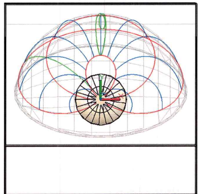
Fig. 2. Bovenaanzicht scaphezonnewijzer.
