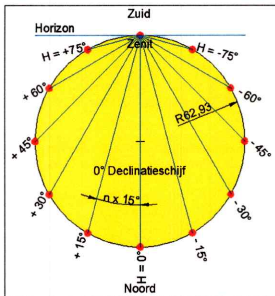
Fig. 5. Uurhoek tussen snijlijn zonnetijdvlakken.
